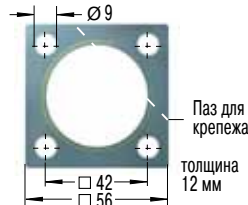
Квадратный фланец
