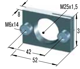
Прямоугольный фланец
