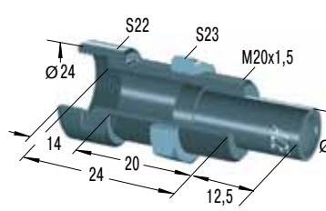
Адаптер боковой нагрузки
