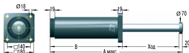
Фронтальная сторона фланца -F
