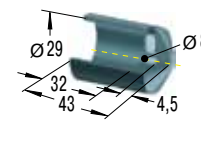
Защитный колпачок
