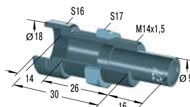
Адаптер боковой нагрузки
