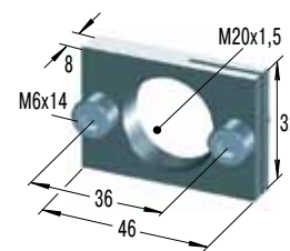
Прямоугольный фланец
