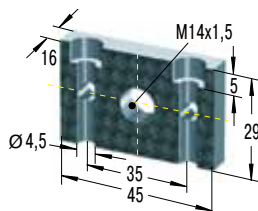
Универсальная опора
