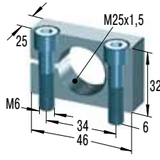
Опора-зажим
