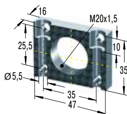
Универсальная опора
