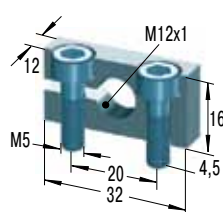
Опора-зажим
