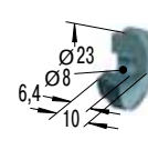
Стальной колпачок
