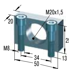
Монтажная опора
