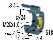
Защитная воздухо-напорная втулка
