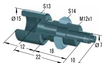
Адаптер боковой нагрузки
