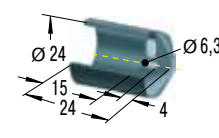
Защитный колпачок
