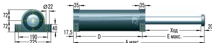
Боковое крепление на кронштейне -S
