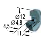
Стальной колпачок
