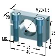
Опора-зажим
