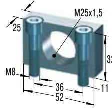
Монтажная опора
