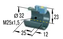
Ограничительная втулка с бесконтактным выключателем
