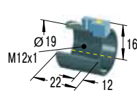
Ограничительная втулка с бесконтактным выключателем
