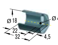
Защитный колпачок
