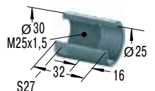
Ограничительная втулка
