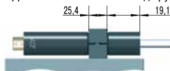
Перегородочное крепление для VC25...F с крепежным блоком KB... (доступен корпус 23,8 мм без резьбы)
