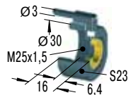
Защитная воздухо-напорная втулка
