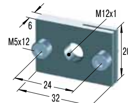
Прямоугольный фланец
