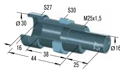
Адаптер боковой нагрузки
