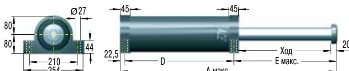
Боковое крепление на кронштейне -S
