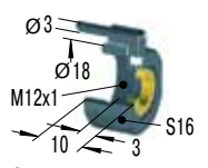
Защитная воздушно-напорная втулка
