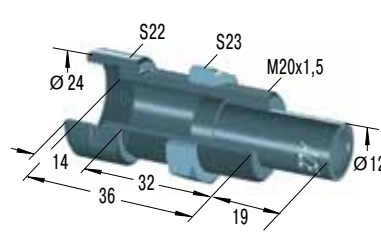
Адаптер боковой нагрузки
