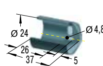
Защитный колпачок
